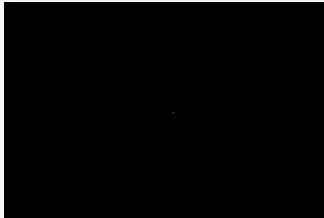
Venus
