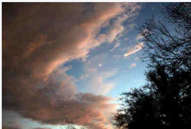
Planet Venus
